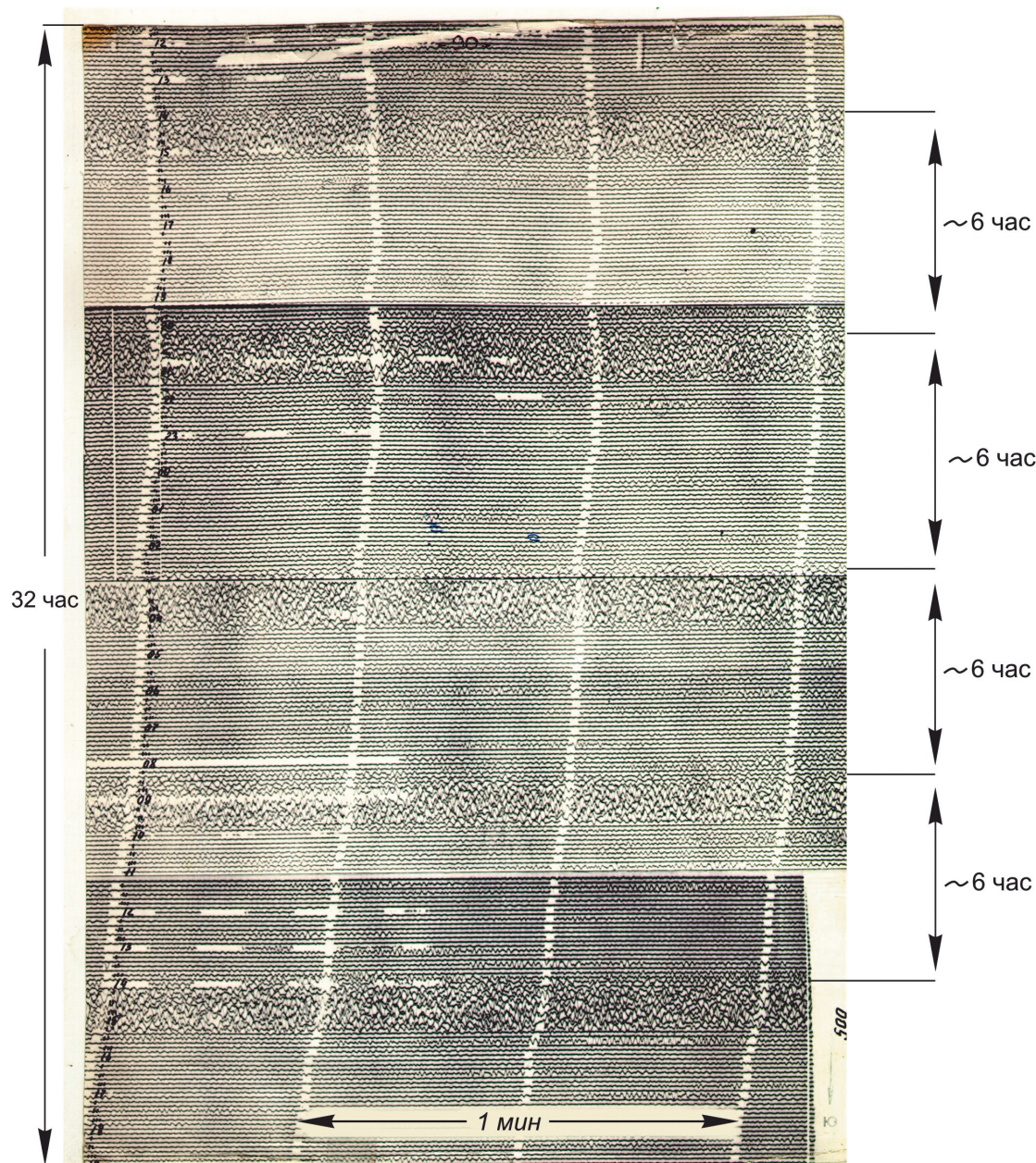
Рис. 2. Фрагменты четырех последовательно записанных сейсмограмм (по 8 часов каждая), зарегистрированных на сеймостанции Апахончич, в 14 км от вершины Ключевского вулкана с 11 ч 37 мин 30 июля по 19 ч 00 мин 31 июля 1984 г. [Ozerov, Konov, 1988]. Темные полосы на сейсмограммах соответствуют интервалам фонтанирования раскаленных бомб ~ 1 ч, светлые – интервалам ослабления взрывной деятельности ~ 5 ч..
