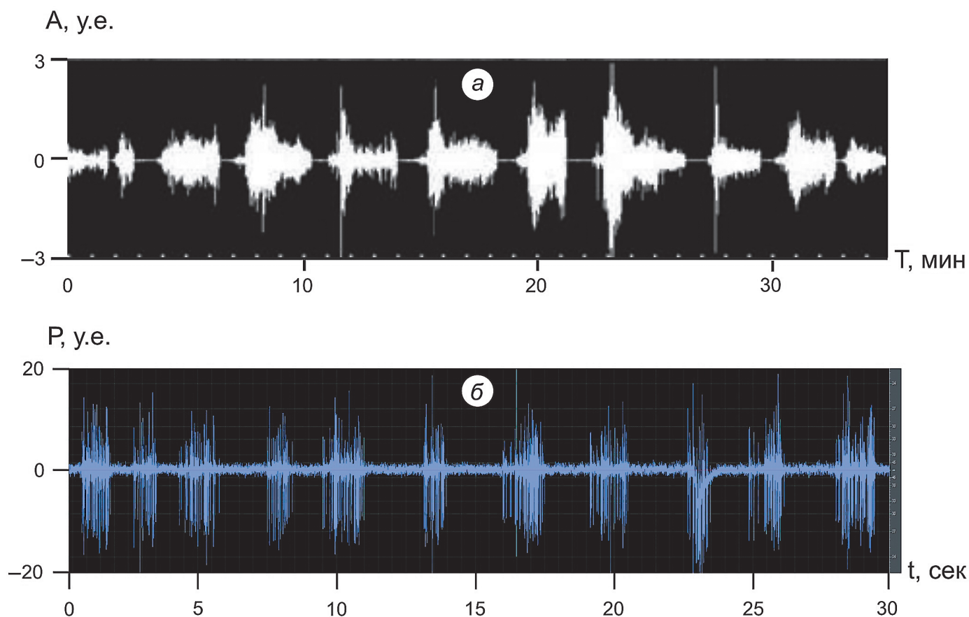
Рис. 5. Сопоставление акустических записей сигнала подводного извержения вулкана NW Rota-1 в Марианской впадине (2006 г.) и сигнала кластерного газогидродинамического режима на поверхности модельной жидкости – по результатам экспериментальных исследований на КАМБИ:
