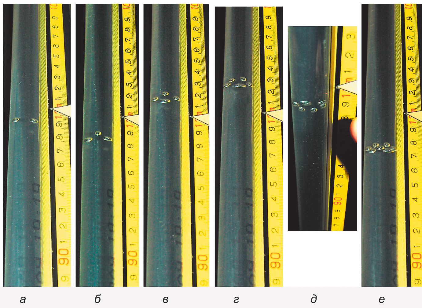
Рис. 8. Неблокированные пузырьковые кластеры с минимальным числом пузырьков в барботажной колонне: а – двухпузырьковый, б – трехпузырьковый, в – четырехпузырьковый, г – пятипузырьковый, д – шестипузырьковый, е – семипузырьковый; все пузырьки одного размера, диаметр ~ 2 мм. Наблюдаемые различия в форме и размерах пузырьков обусловлены искажением за счет изгиба пластикового шланга. Фотографии пузырьковых кластеров выполнены на участке вертикального прозрачного шланга КАМБИ на уровне 13-го метра
